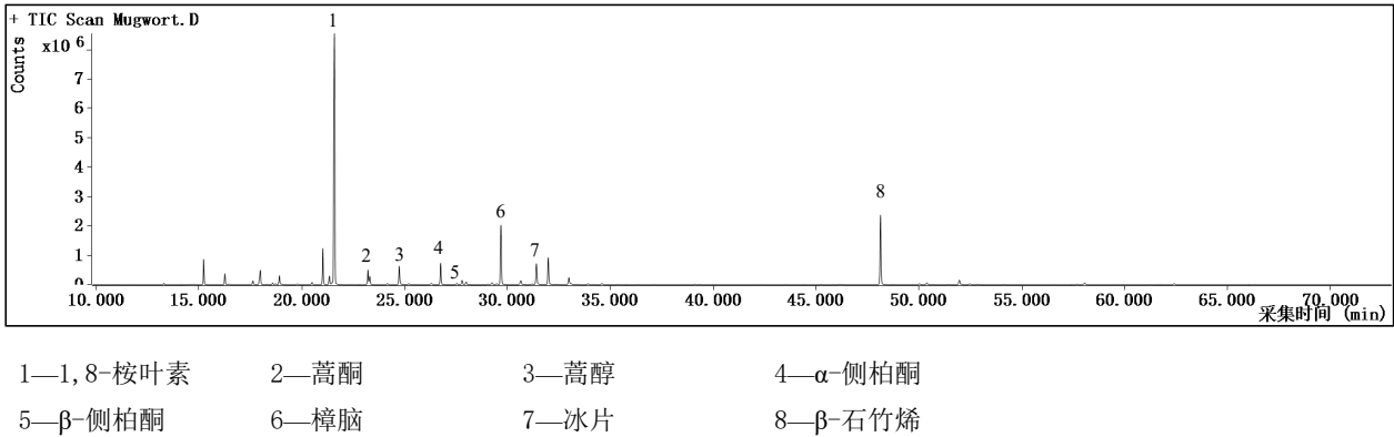
图A.1 艾草精油典型气相色谱-串联质谱图
